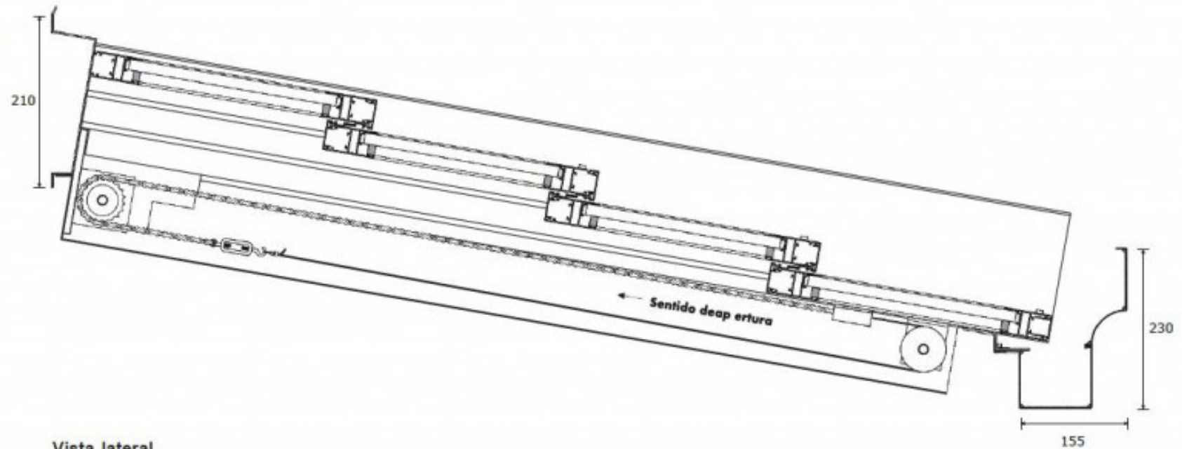
Vista lateral
